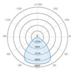
90° Reflector
