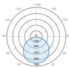
120°, Standard/no Reflector
