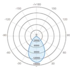
60° Reflector
